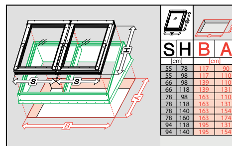
EFW B2/1
