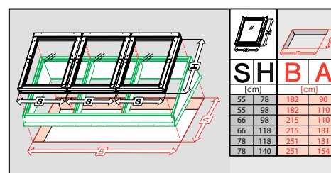
EFW B3/1
