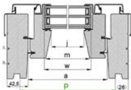
Sponningmaat breedte in mm (p)
