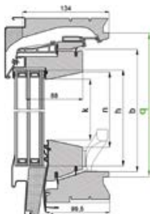
Sponningmaat lengte in mm (q)
